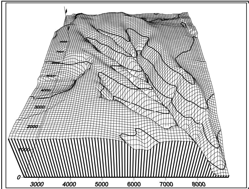
Рис. 1. Трехмерная цифровая модель рельефа верхней части бассейна реки М. Куляльник
