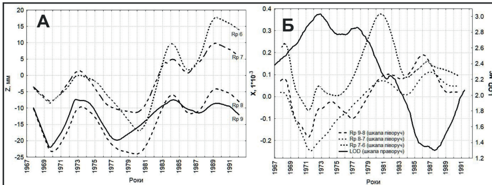
Рис. 3. А – динаміка вертикальних ( Z , мм) і (Б) – горизонтальних відносних деформацій ( X , 1 \cdot 10^{-3} ) ділянок штольні 2 між суміжними реперами (корінна частина масиву порід) за період із 1966 по 1992 рр. На рис. Б також наведено графік параметра LOD ( LOD – швидкість осьового обертання Землі виражена в відхиленні тривалості доби в мс від стандартної – 86400 с)
